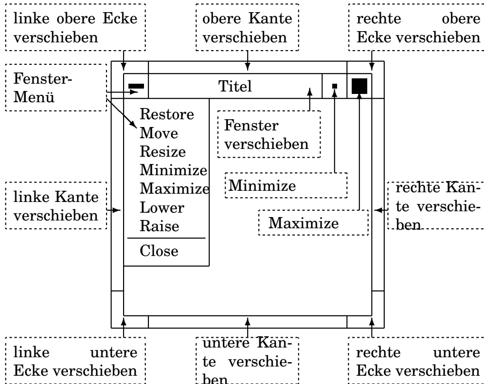
Abb. 2.9: OSF/Motif-Fenster
