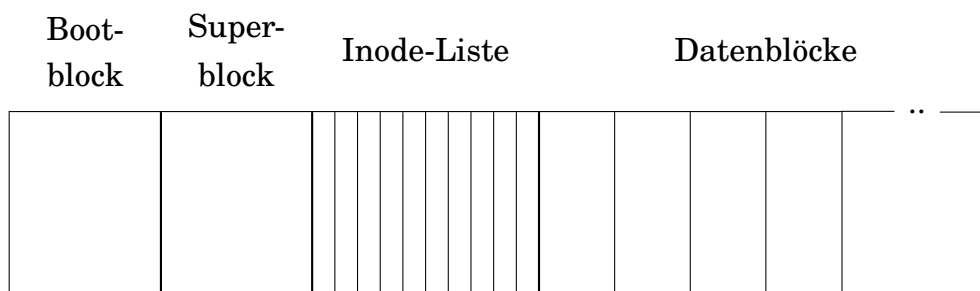
Abb. 2.3: UNIX-Datei-System, Sicht von unten
